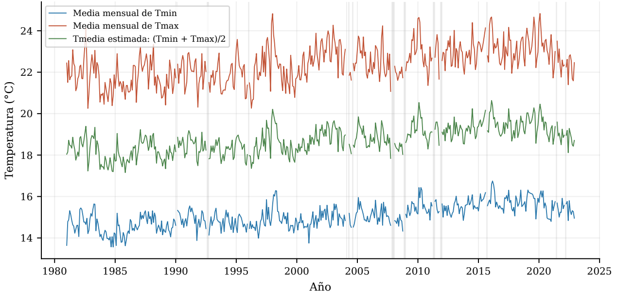
Figura 3: Medias mensuales de Tmin, Tmax y temperatura media estimada de la cuenca.
