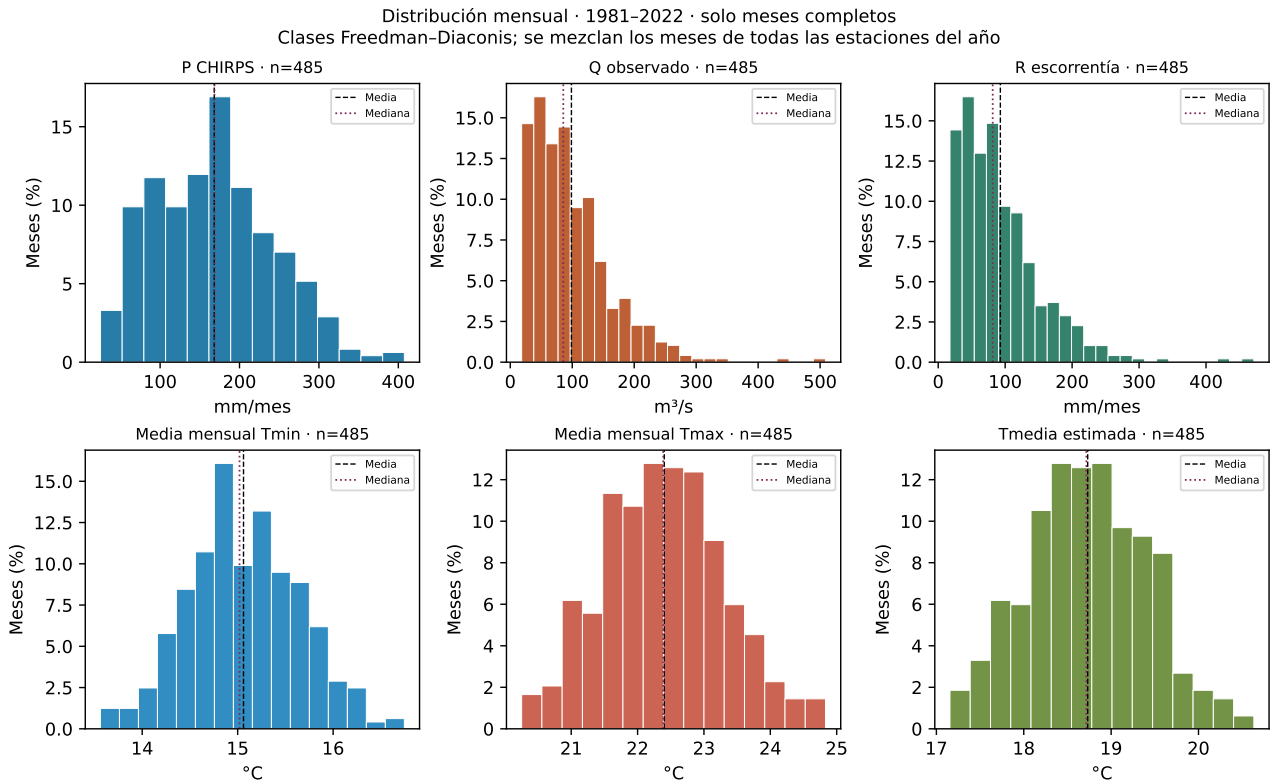
Figura 9: Distribuciones de meses válidos, 1981–2022; unidades indicadas en cada panel.
