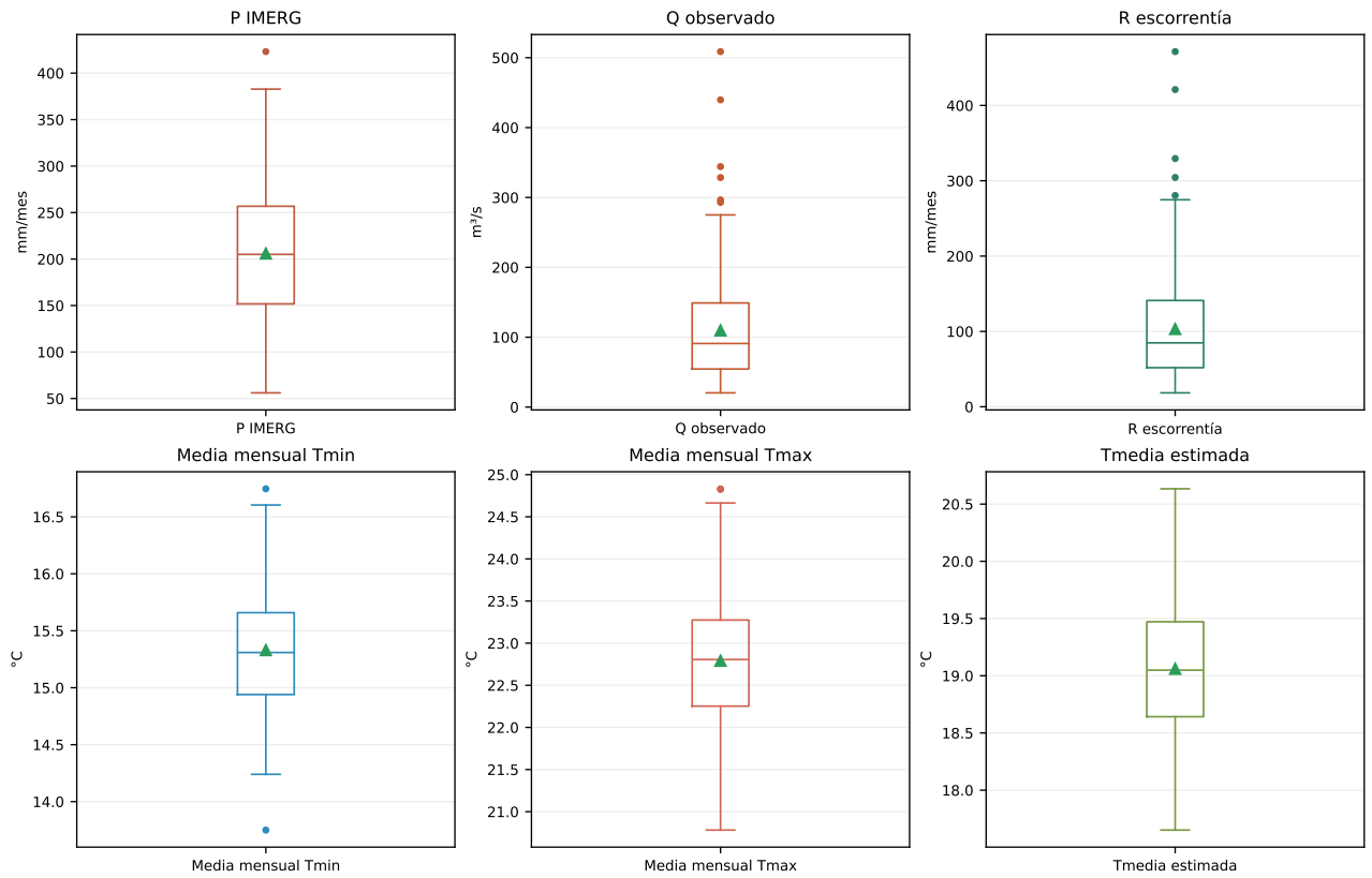
Figura 12: Diagramas de caja comparables del mismo periodo común (n=285).
