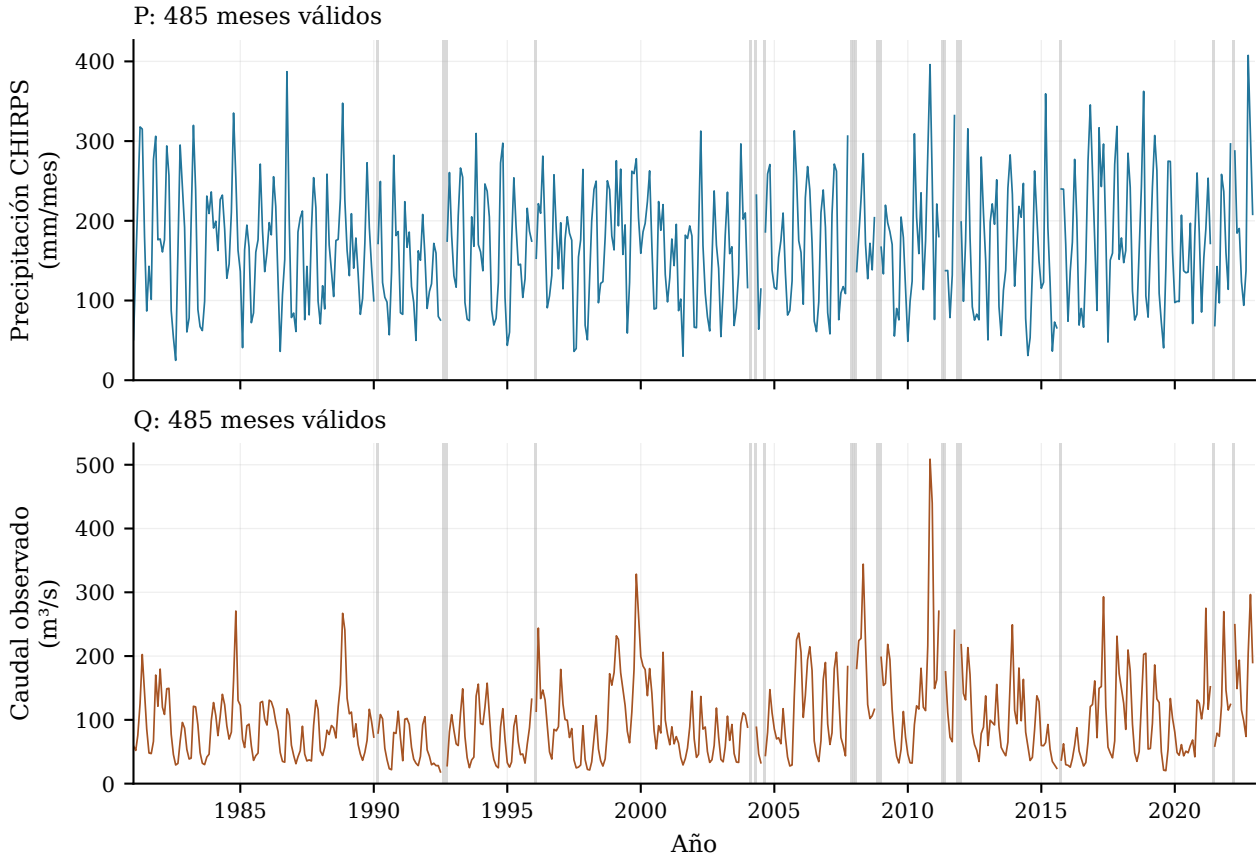
Figura 1: Precipitación acumulada y caudal medio mensuales de La Vieja–Cartago. Los paneles comparten el eje temporal; las franjas grises indican meses excluidos por días faltantes. Elaboración propia con CAMELS-COL.
