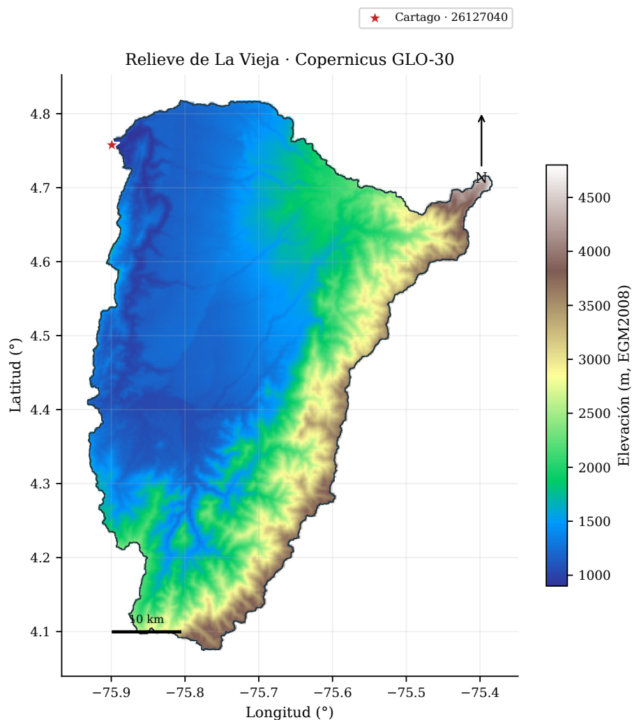
Figura 8: Relieve de La Vieja con Copernicus GLO-30. Alturas en metros, EGM2008.
