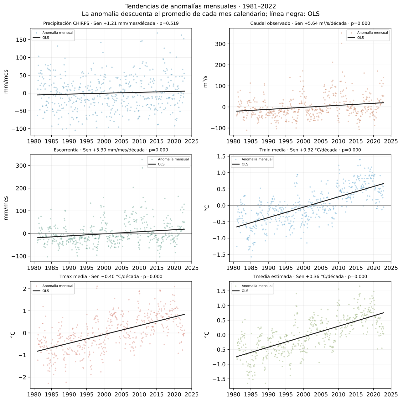
Figura 17: Anomalías mensuales y recta OLS, 1981–2022. Los títulos presentan la pendiente de Sen estacional por década y el valor p de Mann–Kendall estacional.
