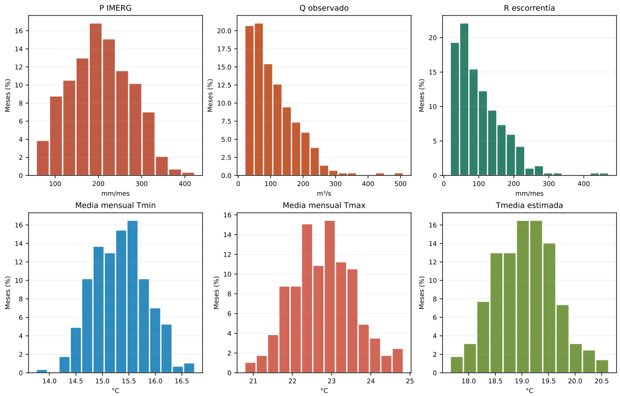
Figura 11: Histogramas comparables del periodo común: IMERG, Q, R, Tmin, Tmax y Tmedia estimada (n=285).
