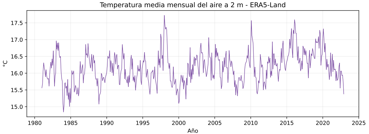
Figura 4: Temperatura media mensual del aire a 2 m de ERA5-Land, promedio ponderado sobre la cuenca de La Vieja, 1981–2022.
