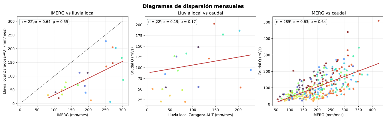
Figura 15: Diagramas de dispersión requeridos. La línea discontinua en IMERG–lluvia local es 1:1.
