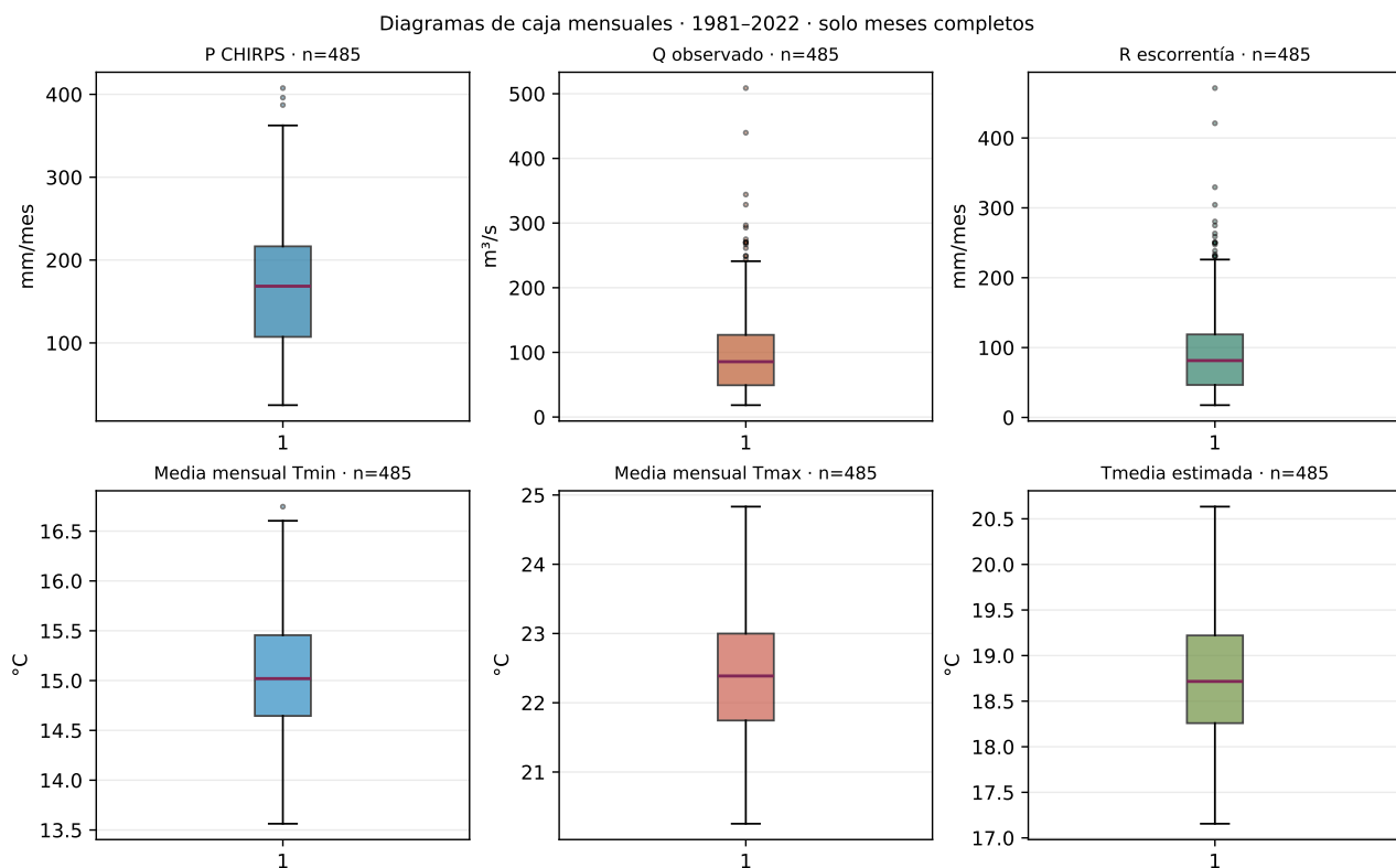
Figura 10: Diagramas de caja de meses válidos. La línea central es la mediana; la caja representa Q1–Q3; los puntos son valores fuera de 1,5 IQR.
