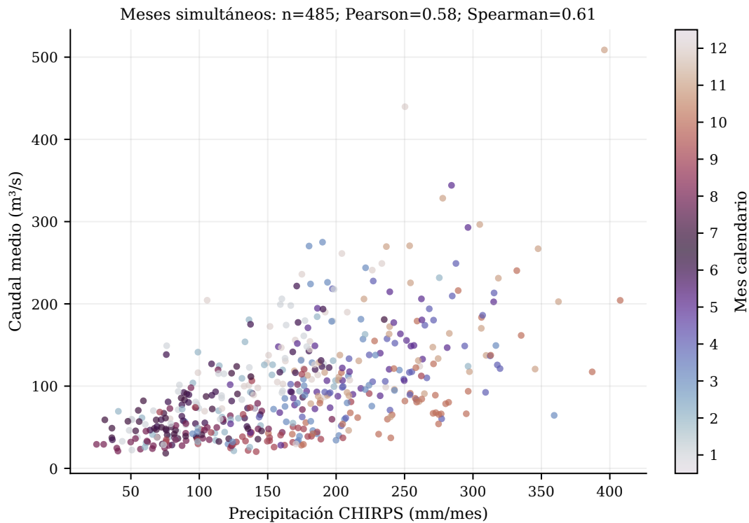
Figura 5: Relación descriptiva entre precipitación CHIRPS y caudal, sin rezago.
