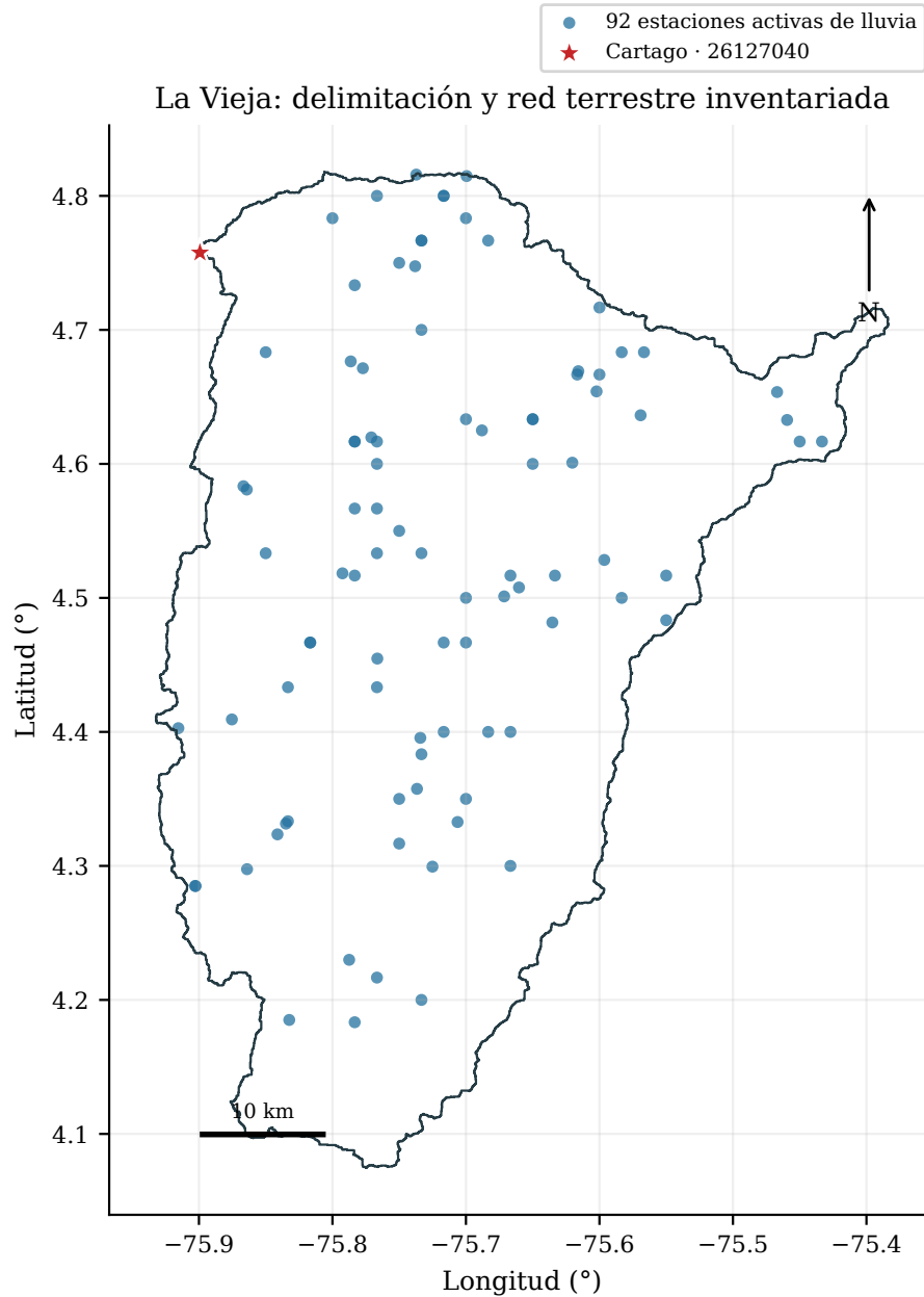
Figura 7: Cuenca La Vieja hasta Cartago y estaciones terrestres inventariadas.
